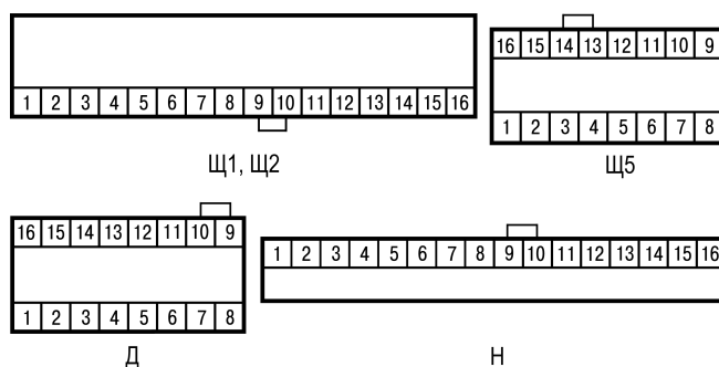
Рисунок 7.8 – Установка переключки
