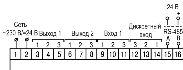
Рисунок 5.7 – Общая схема подключения TRM10–Н
