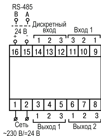
Рисунок 5.6 – Общая схема подключения TRM10–Д
