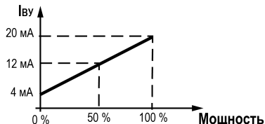
Рисунок 7.6 – Мощность аналогового ВУ
